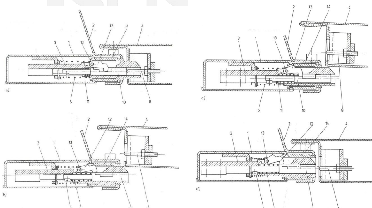
Obr. 3.6 - Dveřní uzávěrka DU4
